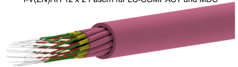
I-V(ZN)HH 12 x 2 Fasern für LC-COMPACT und MDC
