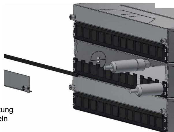
Die Rückwand-Blindabdeckungen am 2, 3 und 5 HE Gehäuse können zur komfortablen Nachrüstung und Wartung von Trunkkabeln mittels ihrer unverlierbaren Schrauben abgenommen werden.
