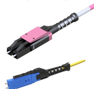
MDC Stecker für Mega High Density (MHD)
